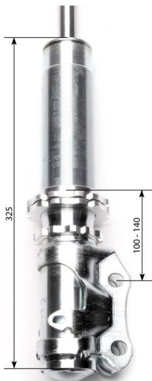
Fahrwerk Achse 1
